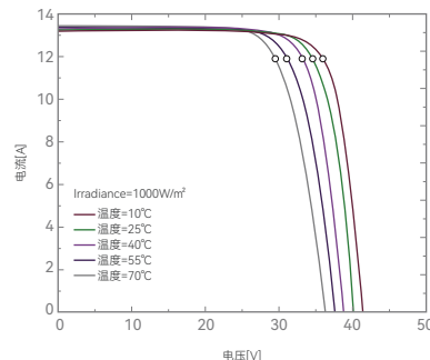
不同电池温度下电流-电压曲线图
